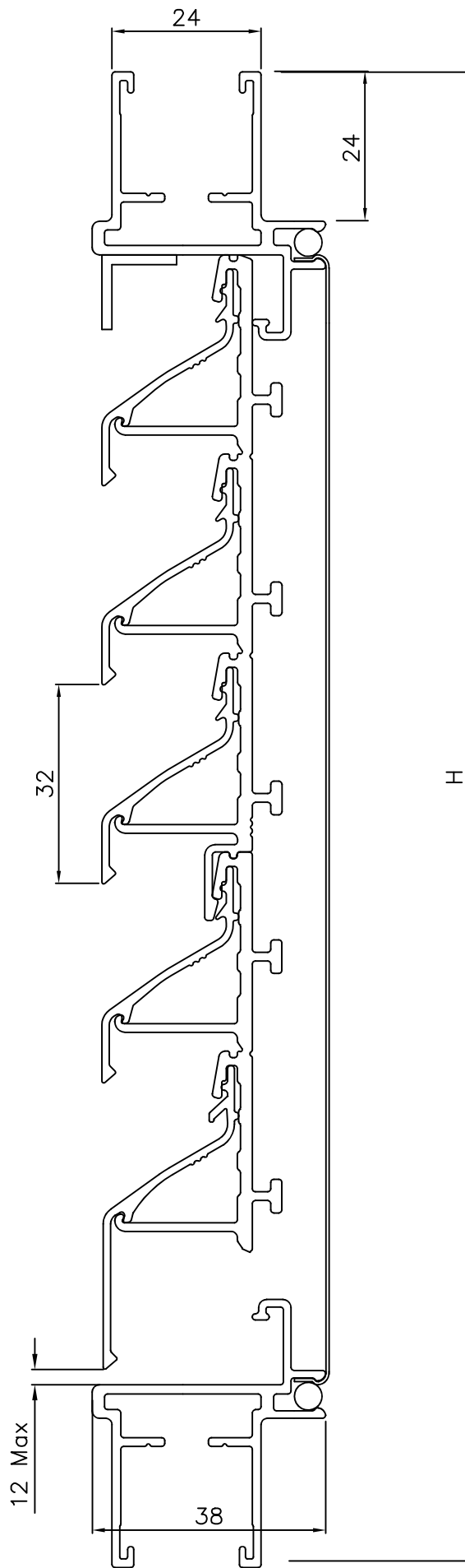
AVS32GL24 Vertical Section 1:1
